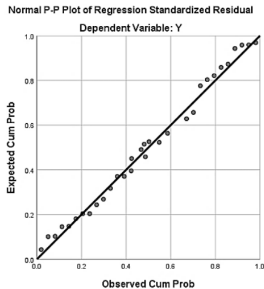
Gambar 1 Normalitas Data
