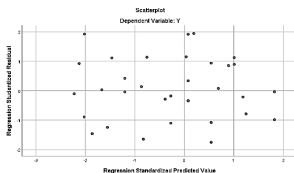
Gambar 2 Heteroskedastisitas
