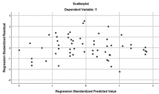
Gambar 2. Tes Heteroskedastisitas
