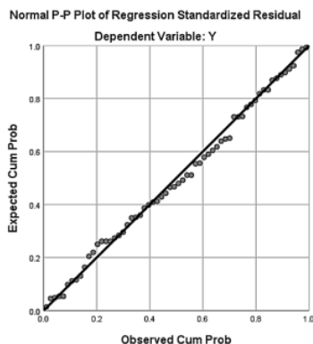
Gambar 1. Tes Normalitas
