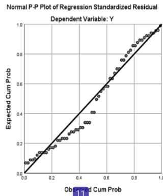
Gambar 1. Uji Normalitas
