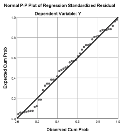
Gambar 2. Normality Plot Sumber hasil olah SPSS
