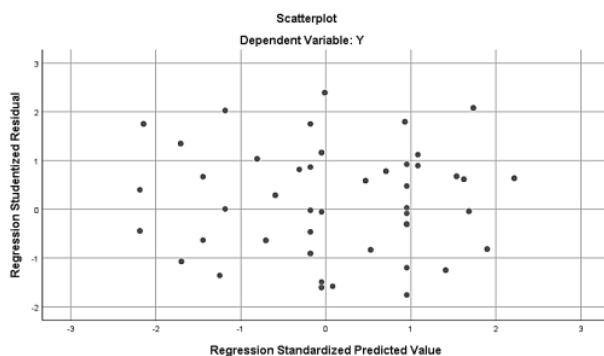
Gambar 3. Scatterplot Dependent Variable Sumber hasil olah SPSS
